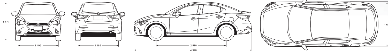
DIMENSIONES (mm) VERSIÓN SEDÁN
